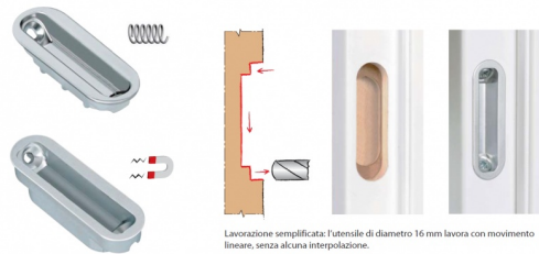
Lavorazione semplificata: l'utensile di diametro 16 mm lavora con movimento lineare, senza alcuna interpolazione.
